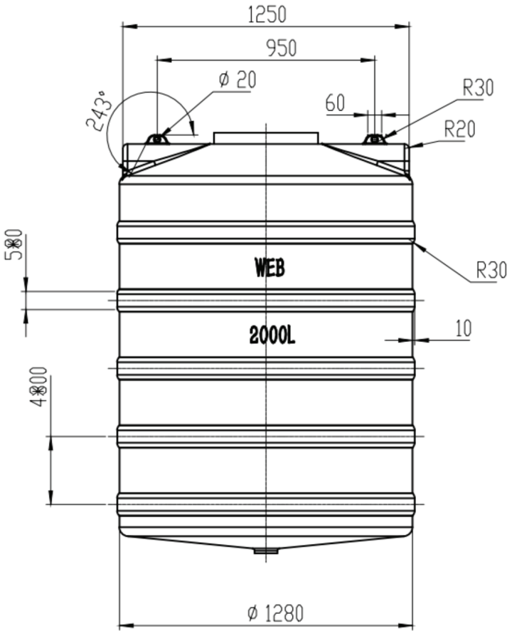
Medidas tanque 2000 lts.
