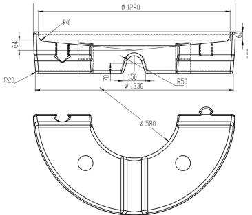
Medidas base para tanque 1100lts y 2000lts.
