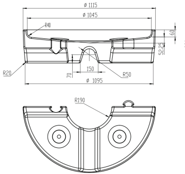
Medidas base para tanque 1100lts y 2000lts.
